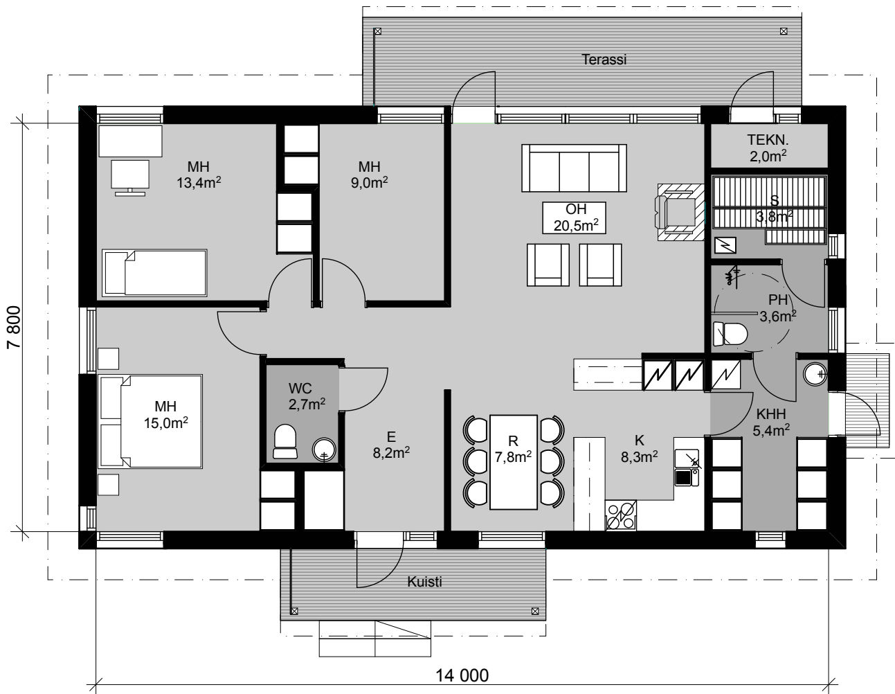
POHJAPIIROS 1:100
